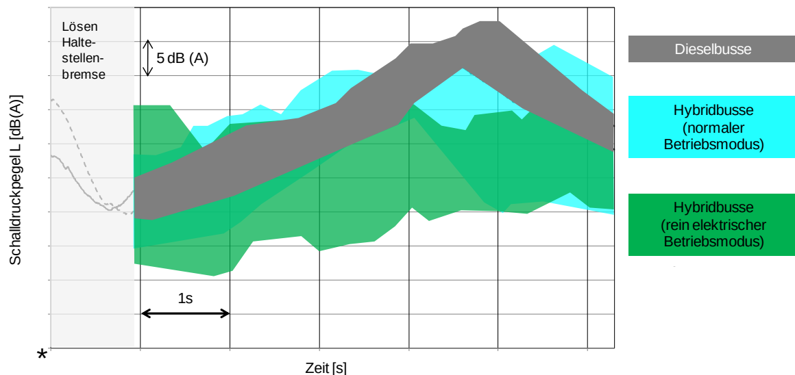
Abbildung 31 Haltestellenabfahrt unter Vollastbedingungen 13
