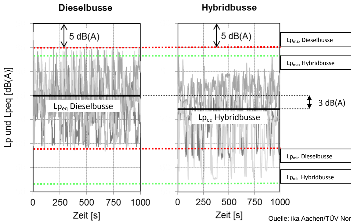
Abbildung 33 Streuband Linienfahrten und Mittelwertpegel: Dieselbusse vs. Hybridbusse
