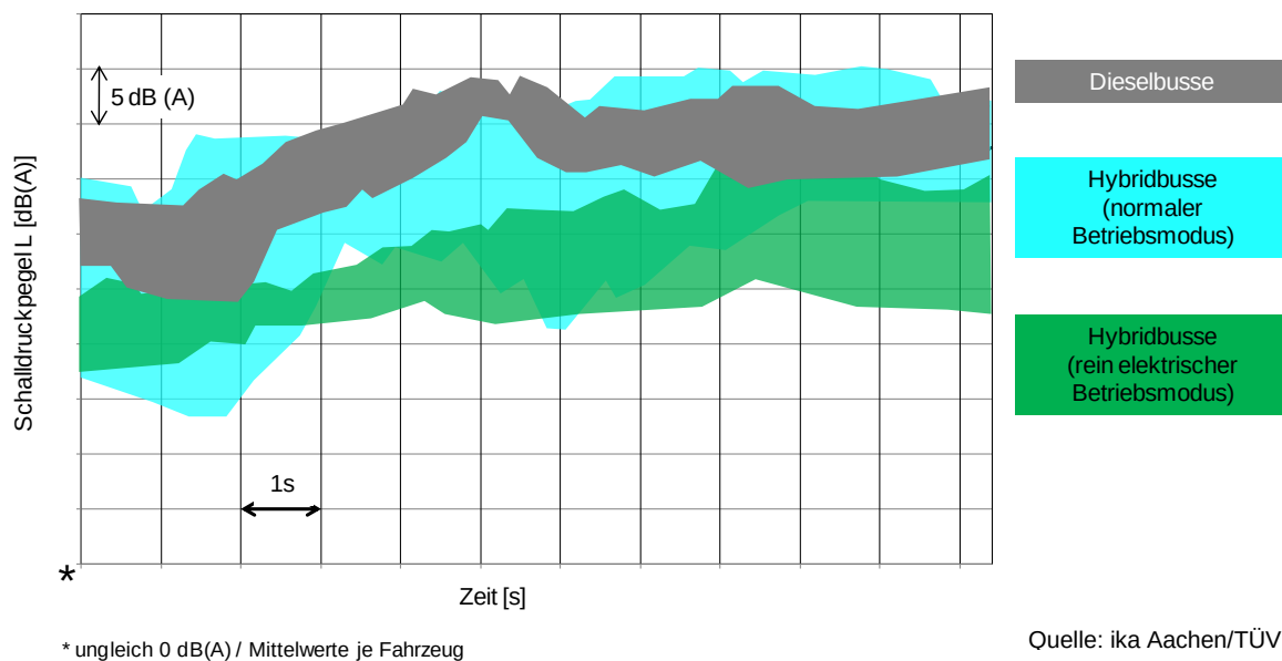
Abbildung 30 Haltestellenabfahrt unter Vollastbedingungen 12
