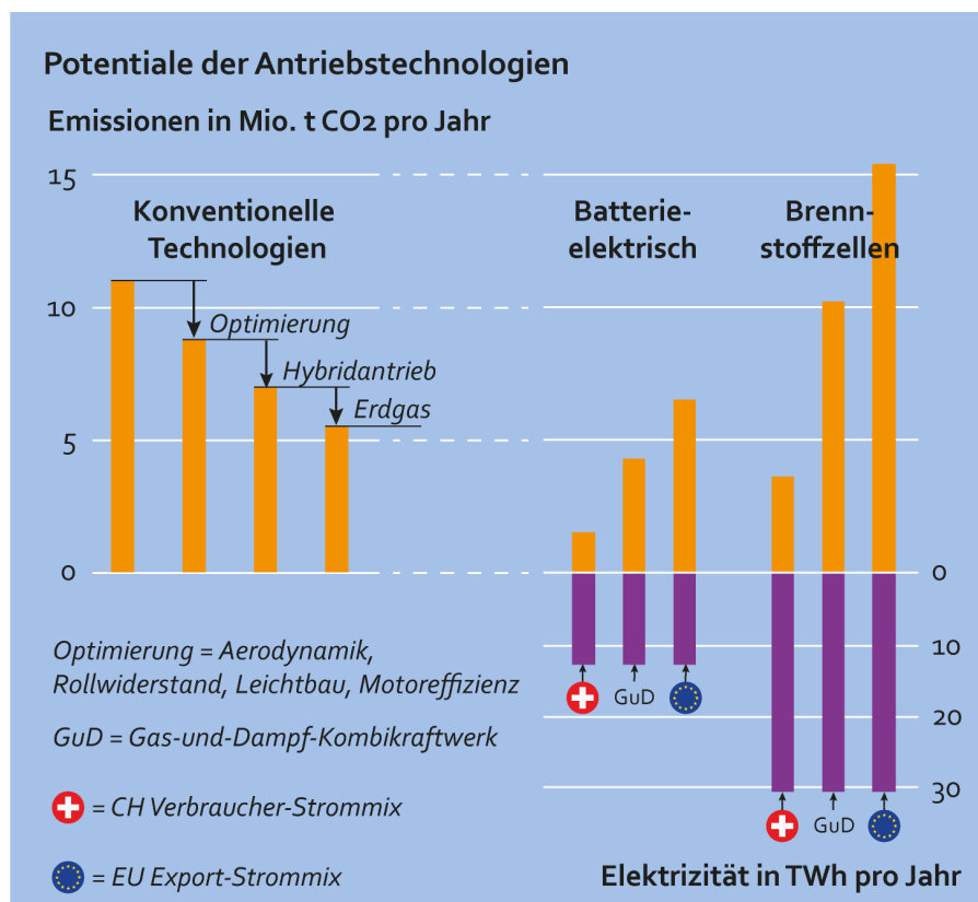
Abbildung 7. Optimierung und erhöhter Einsatz von CO 2 -neutraleren konventionellen Technologien kann schon mehr als 50% CO 2 einsparen. Der CO 2 -Fussabdruck systemverändernder Technologien (batterieelektrisch und Brennstoffzellen) hängt stark von der Stromquelle ab. Der geschätzte durchschnittliche CO 2 -Emissionswert des EU Export-Strommixes beruht auf Daten aus dem Jahr 2014 (Messmer & Fischknecht 2016).
